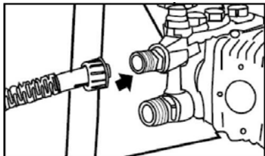
Étape 4:Connecter le flexible au raccord de sortie d'eau du nettoyeur haute pression.
